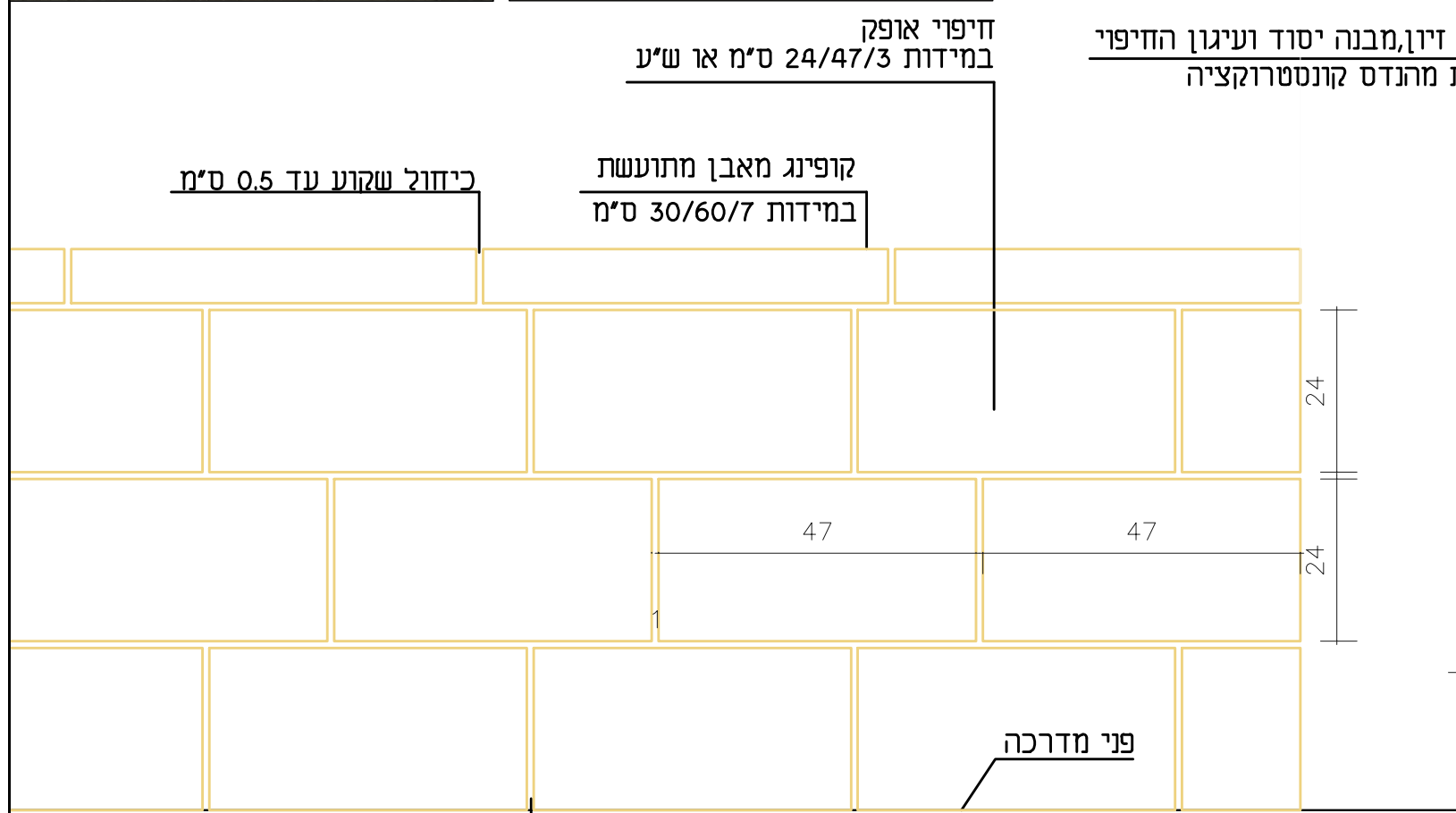
חזית - חיפוי בנדבכים 1 : 10
