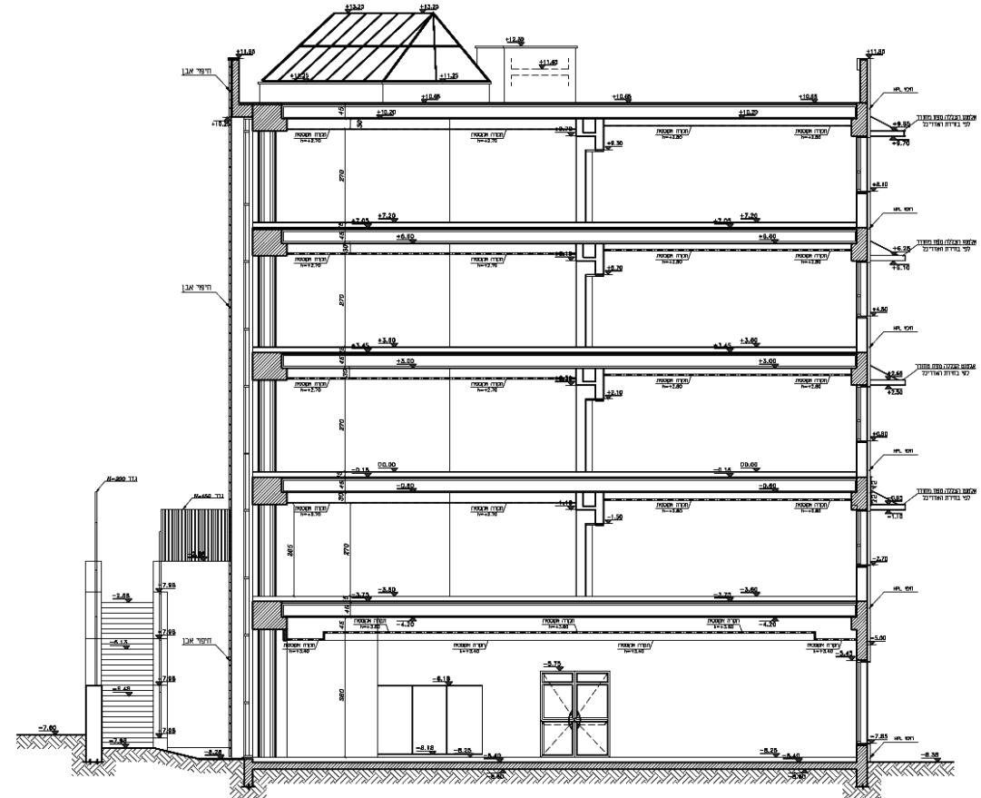
חתך ט-ט
