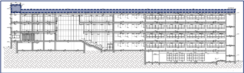
חתך ג-ג לב"ס המתכנן
