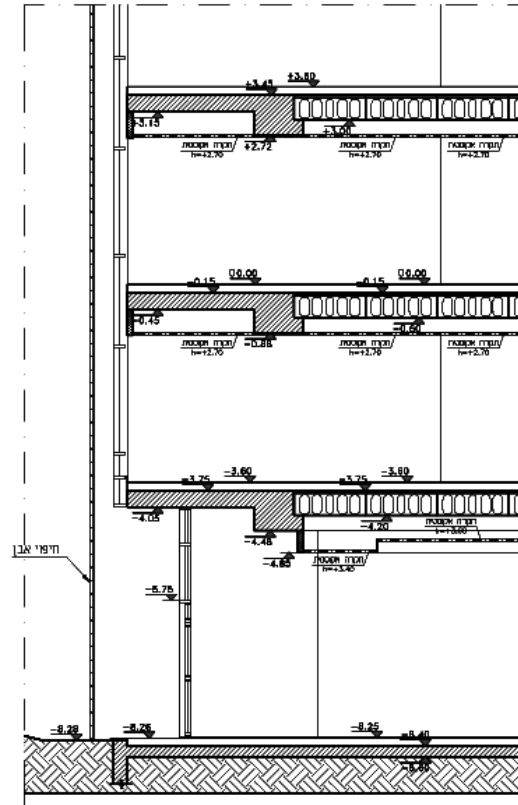
חתך י-י
