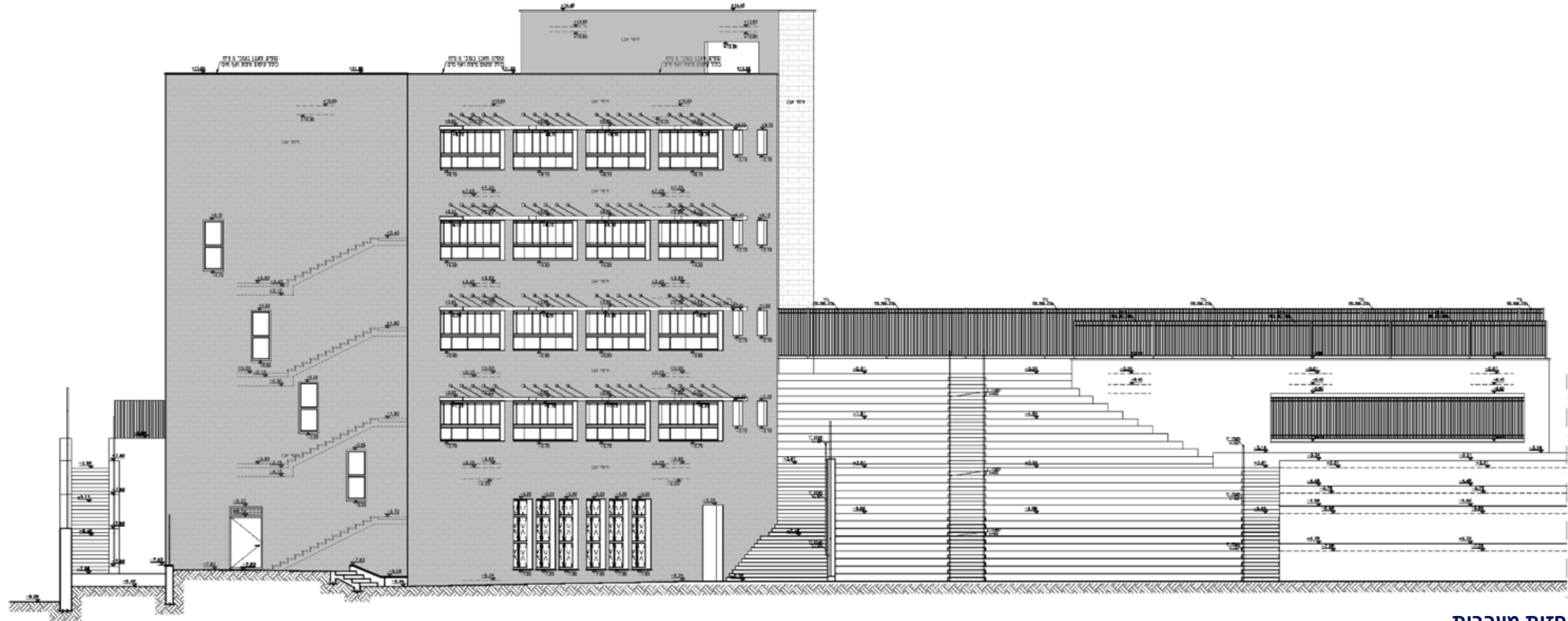
חזית מערבית
