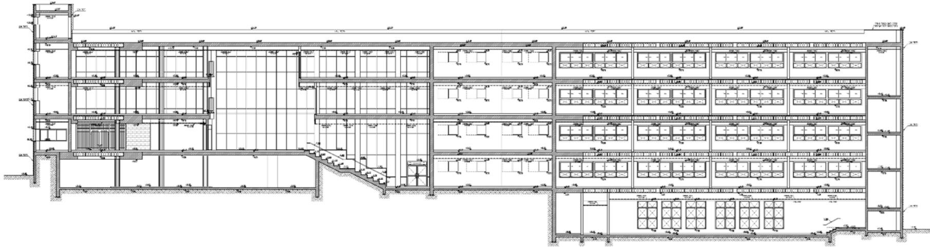
חתך ג-ג
